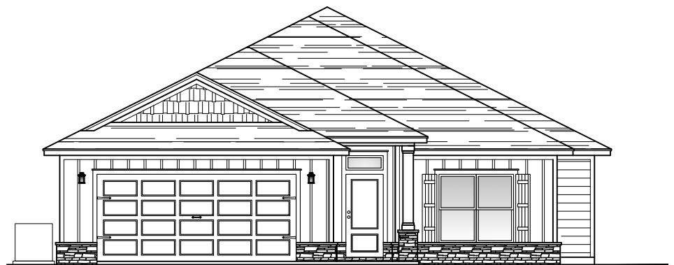
ELEVATION "C"
